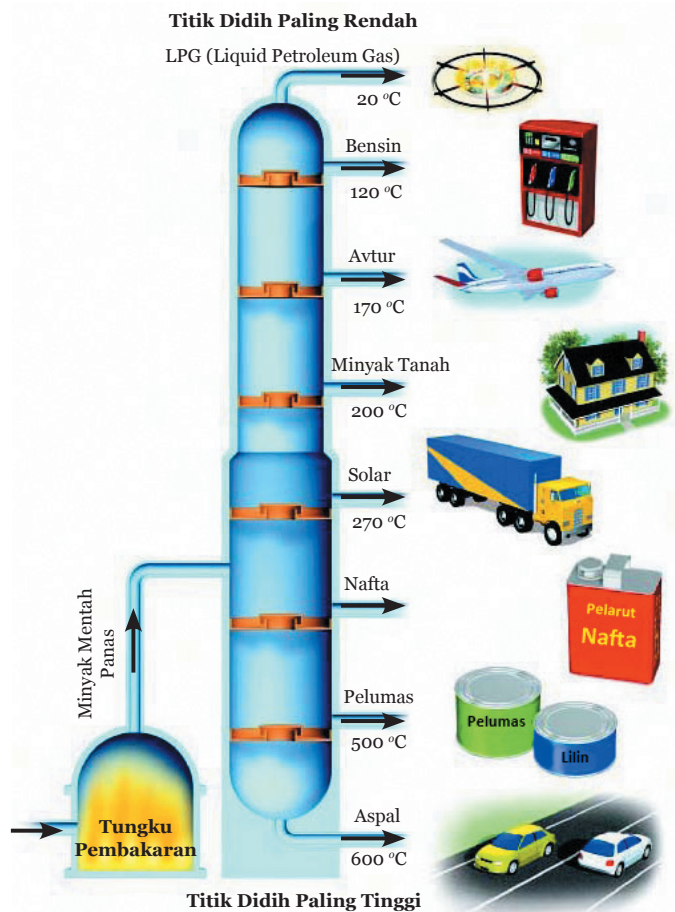
Gambar 10.27 Penyulingan (Distilasi) Minyak Bumi
