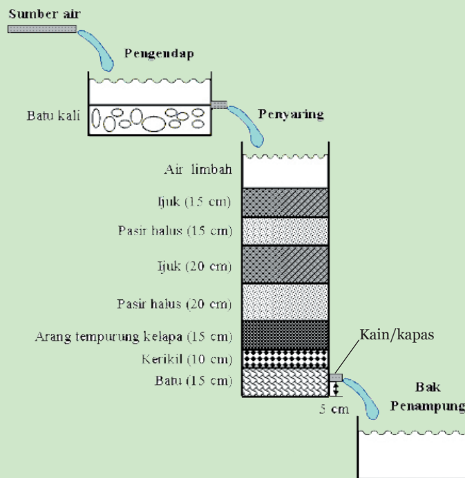
Gambar 10.21 Skema Teknologi Pemurnian Air Sederhana
