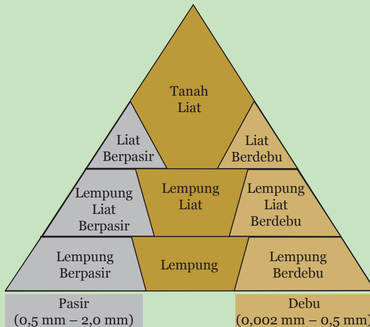
Gambar 9.8 Klasifikasi Tekstur Tanah Berdasarkan Ukuran Butiran Penyusun
