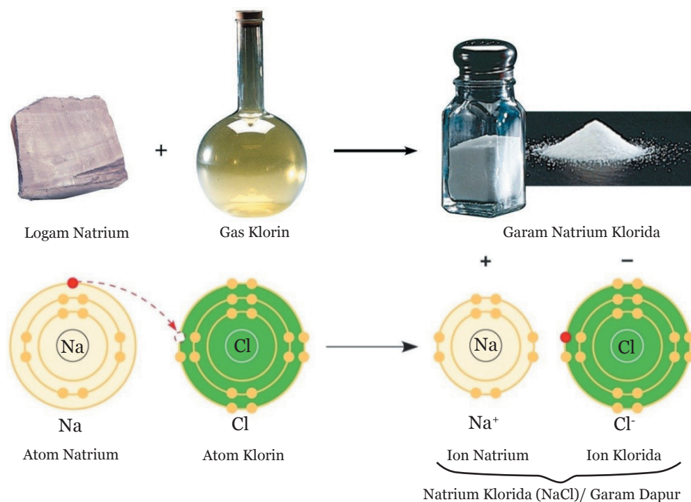
Gambar 8.18 Serah Terima Elektron pada Pembentukan Garam Dapur ( \text{NaCl} )
