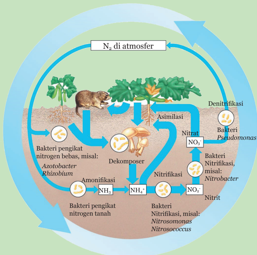
Gambar 8.3 Siklus Nitrogen
