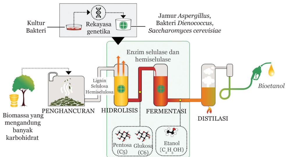
Gambar 10.5 Skema Pembuatan Bioetanol
