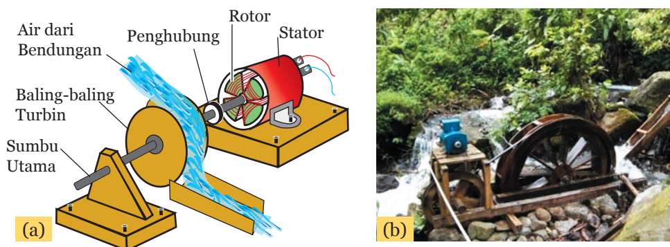
Gambar 10.9 (a) Skema Pembangkit Listrik Sederhana Tenaga Air, (b) Pembangkit Listrik yang Telah diterapkan di Masyarakat
