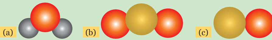
Gambar 8.8 Model Molekul Dalton untuk (a) Air ( H_2O ), (b) Karbon Dioksida ( CO_2 ), (c) Karbon Monoksida ( CO )
