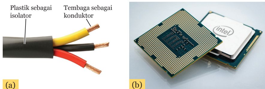
Sumber: (a) quincaileriebeta.com, (b) www.comsol.com Gambar 4.31 (a) Kabel Tembaga sebagai Konduktor dengan Plastik sebagai Isolatornya, (b) Prosesor Komputer Terbuat dari Bahan Semikonduktor
